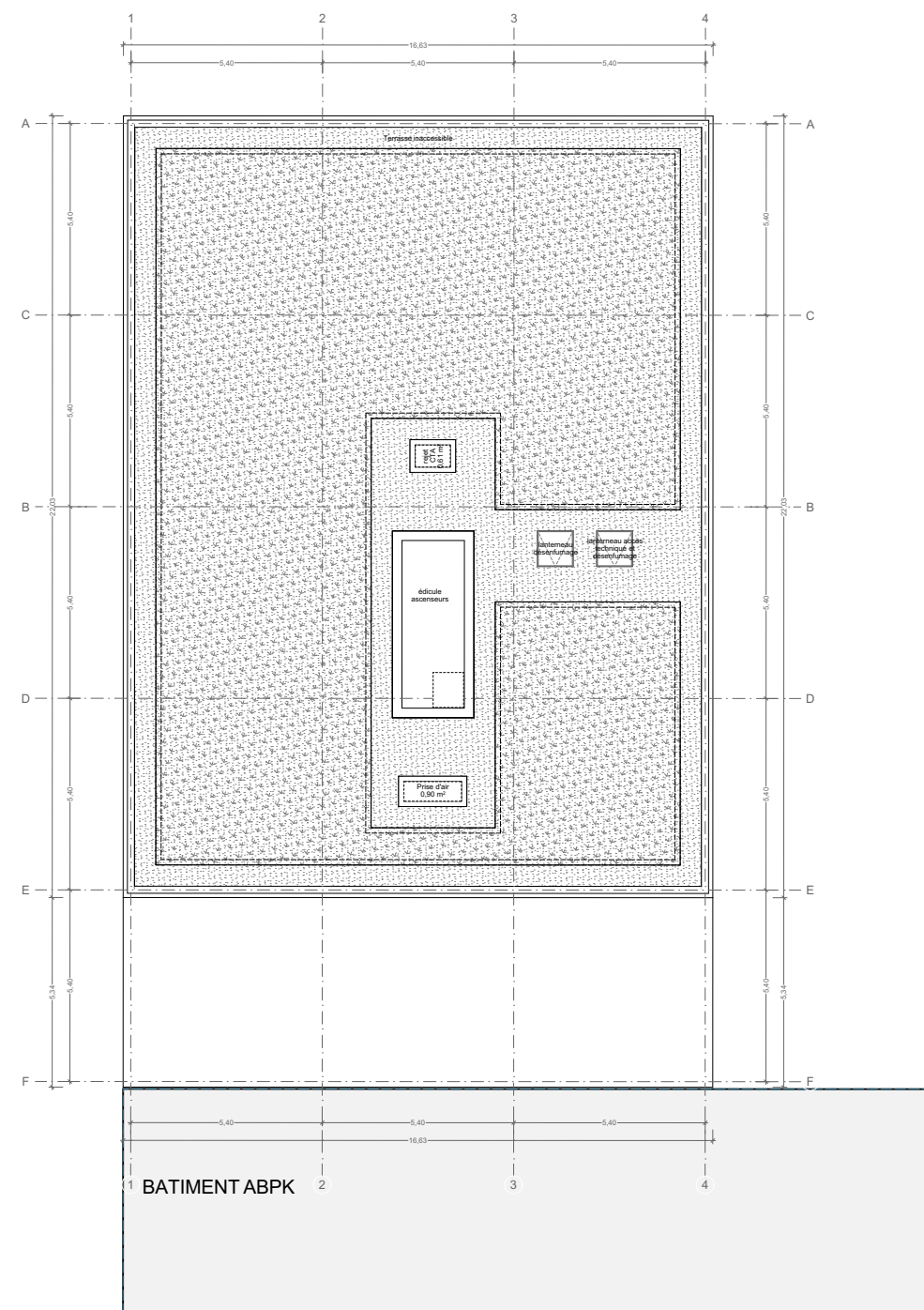
PLAN TOITURE
