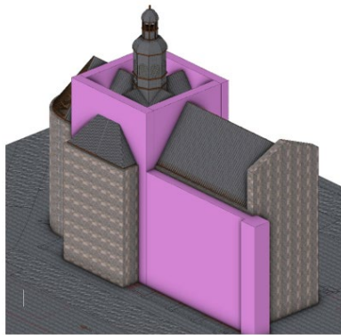
1 - Pose de l'échafaudage périphérique
